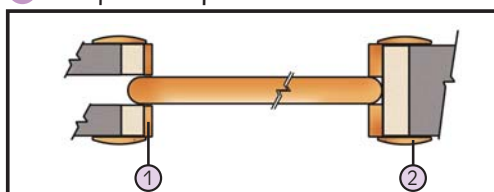
△ Corredera oculta entre tabiques
