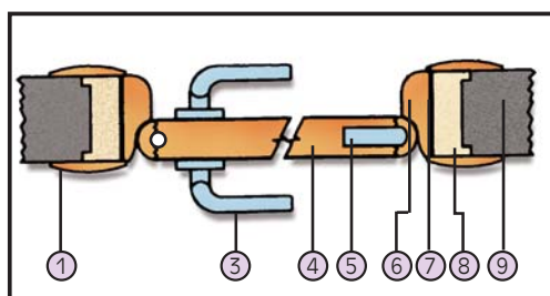
Puerta PIVOTAN sencilla
