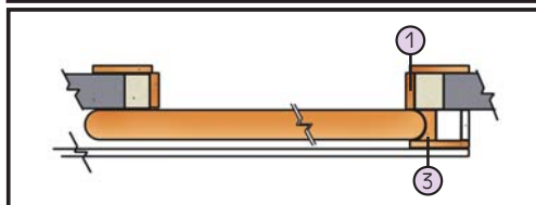
△ Corredera solapada
