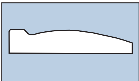
Motllura MOD. 431 80x15mm.
