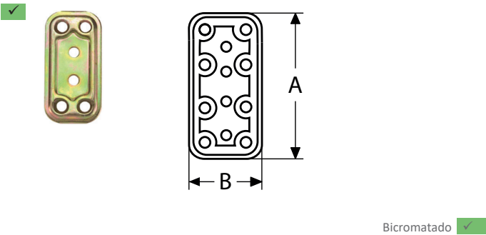
748 JUNTA PLANA
