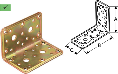
777 JUNTA ANGULAR
