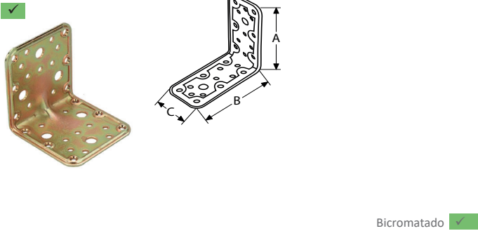
769 JUNTA ANGULAR
