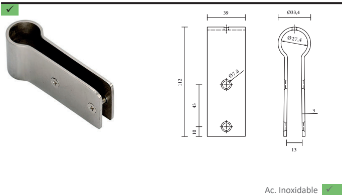
PINZA SUJECCIÓN
