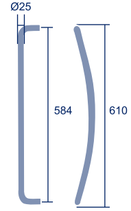
Tirador tubular curvo Con roseta. Referencia: TC/610R Código: 21386
