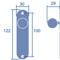
Tirador armario Referencia: I017 Código: 25945 20 udes.
