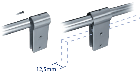
Soporte superior 50mm Referencia: EM002 Código: 23217 Soporte superior 40mm Referencia: EM002-B Código: 26503 7 udes.
